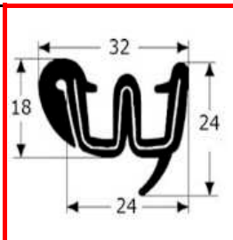
GU400 Unidad
